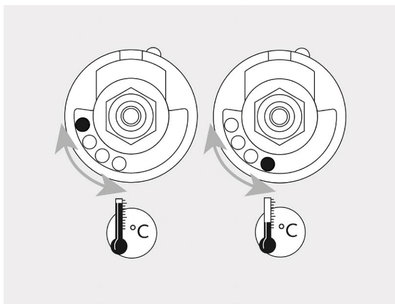
Bild 2 • Beispiel für einen Sicherheitsanschlag zur Temperaturbegrenzung in einer Selbstschlussarmatur von Schell
